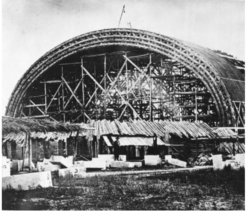
Das Tabernakel, wie es während des Baus und nach der Fertigstellung aussah. Die einzigartige „Eierschalen“-Konstruktion ergab sich aus großen, brückenartigen Trägern, die das 46 m breite Gebäude überspannten. Es ist 24 m hoch und 76 m lang.
