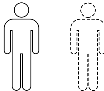
Fysisk legeme
